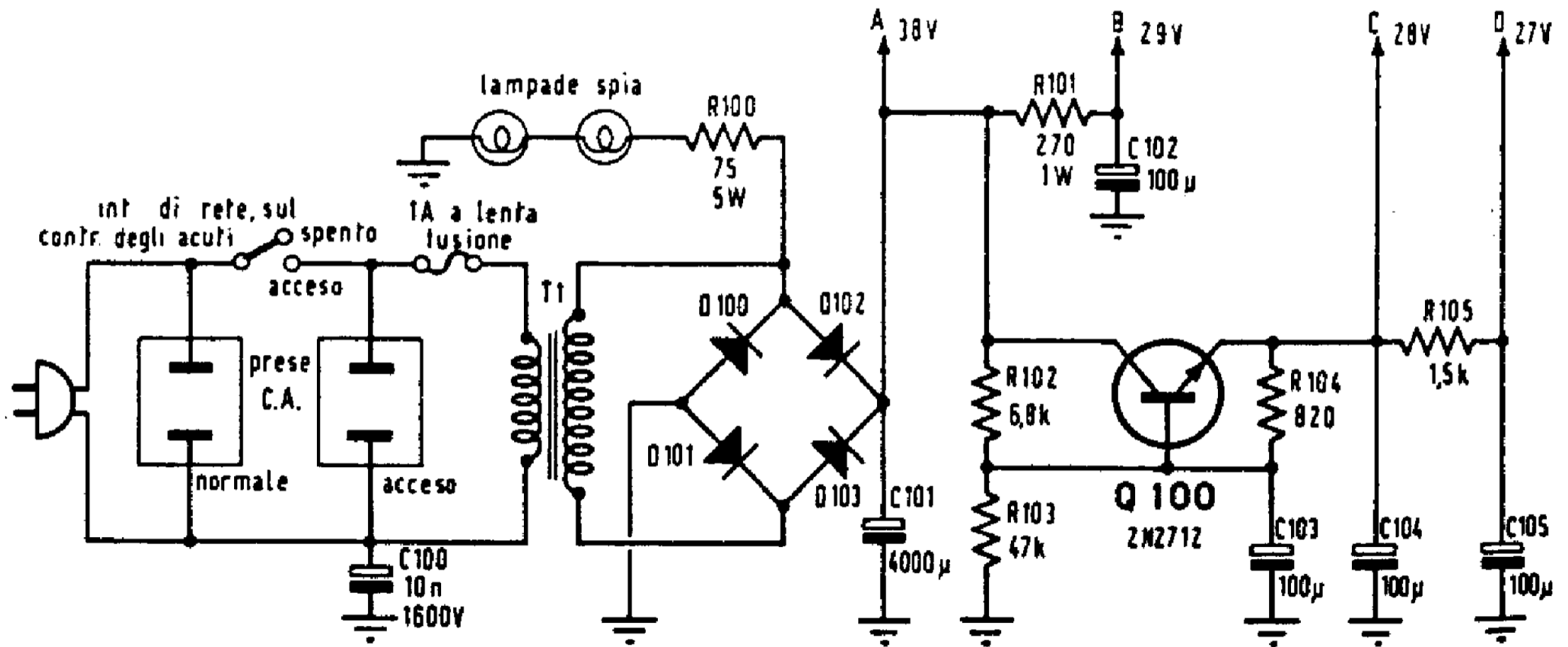
- Schema elettrico dell'alimentatore.
